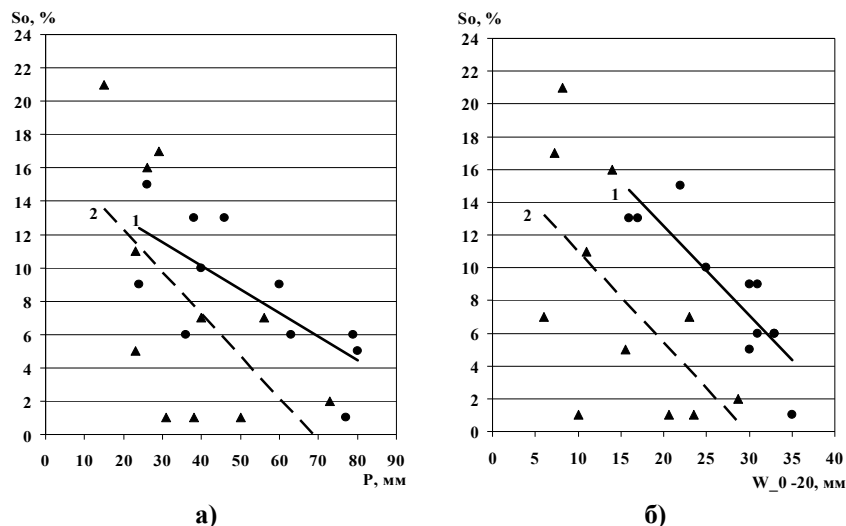
Рис. 7. Зависимость величины S_0 от количества осадков (а) и запасов продуктивной влаги (б) в пахотном слое почвы за третью декаду августа – первую-вторую декады сентября по Республике Татарстан (1) и Оренбургской области (2).
