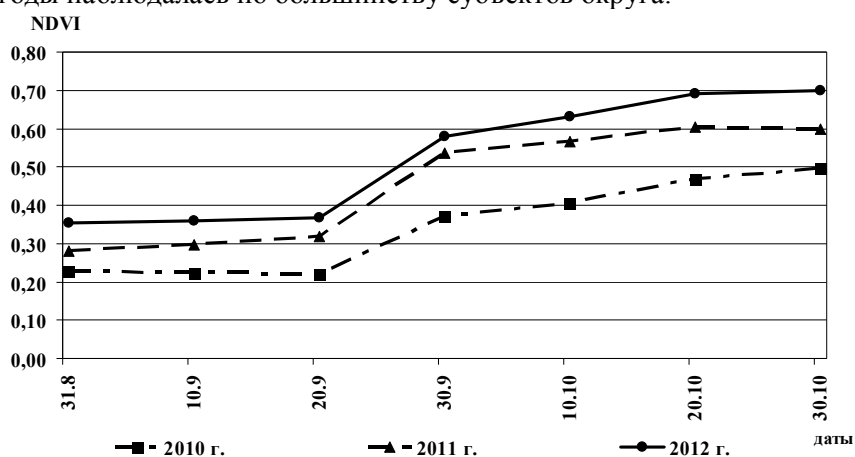
Рис. 5. Динамика NDVI по Саратовской области за 2010–2012 гг.
