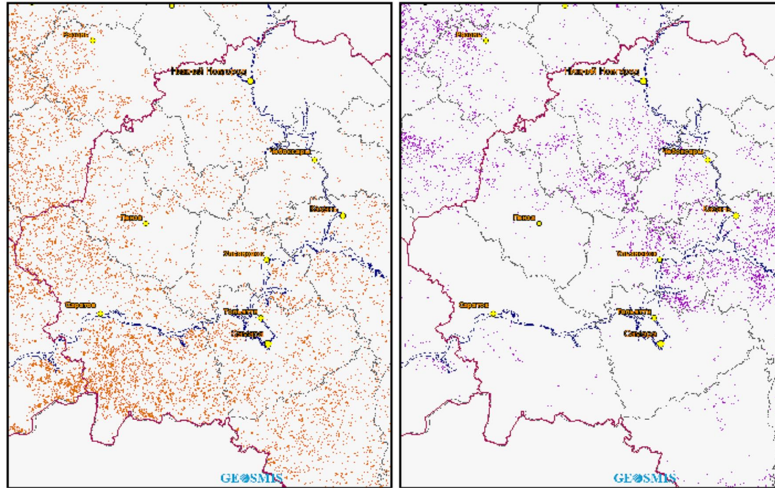
Рис. 3. Примеры выявленных по спутниковым данным посевов озимых культур осенью в конце вегетации в Приволжском федеральном округе при благоприятных (сезон 2011–2012 гг., слева) и неблагоприятных (сезон 2010–2011 гг., справа) условиях развития посевов.
