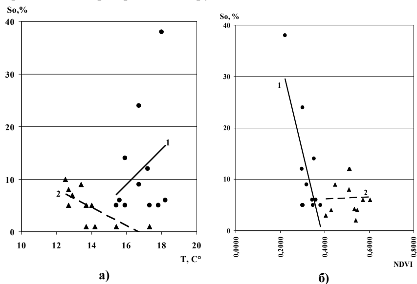
Рис. 8. Зависимость величины S_0 от температуры воздуха за третью декаду августа – вторую декады сентября в Саратовской (1) и Нижегородской (2) областях (а); от NDVI в Саратовской (1) и Кировской (2) областях (б).
