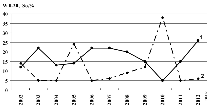
Рис. 2. Динамика запасов продуктивной влаги (1) в пахотном слое почвы ( W_{0-20} ) и площадей озимых зерновых культур (2) в плохом состоянии осенью ( S_0 ) по Саратовской области за 2002–2012 гг.
